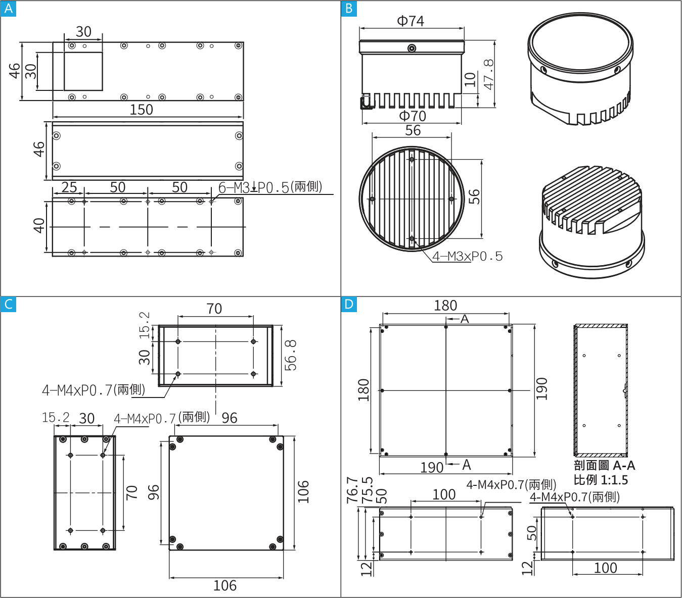
尺寸圖
