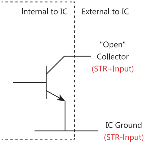
*Open Collector 形式接法說明
