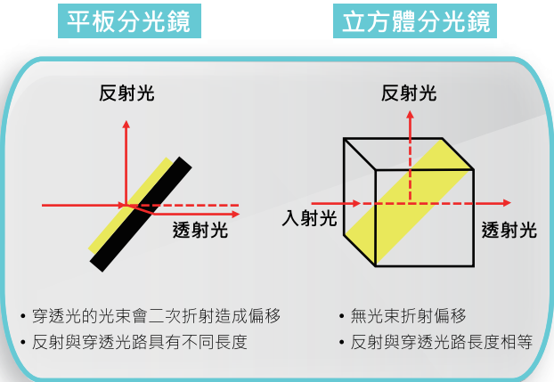
一般外同軸 (平板分光鏡) 稜鏡版外同軸 (立方體分光鏡)
