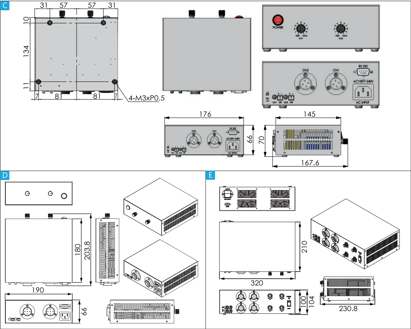
尺寸圖
