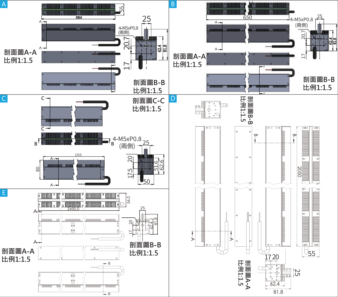
尺寸圖
