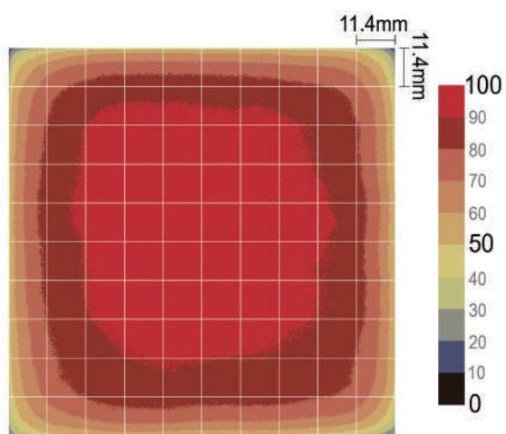
實驗產品:BL-100100 (13mm厚)
